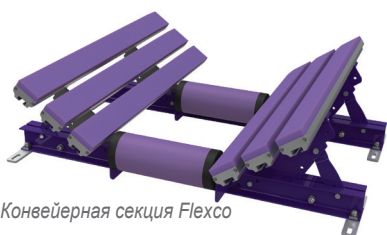
Конвейерная секция Flexco® со скатами и амортизирующими роликами CoreTech (EZSB-I)
