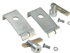
Комплект крепежа Bolt-On PAL PAK
